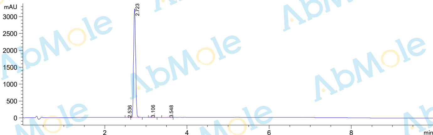
DAD1 A, Sig=214,4 Ref=off
